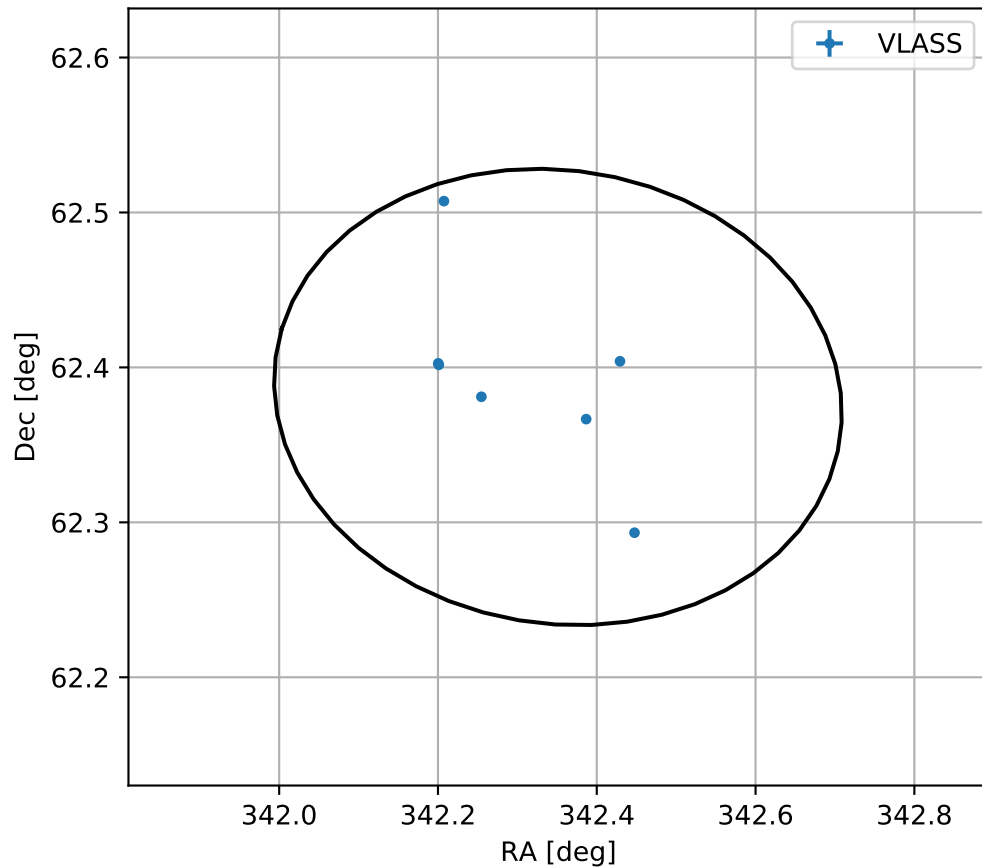
4FGL J2249.4+6222
