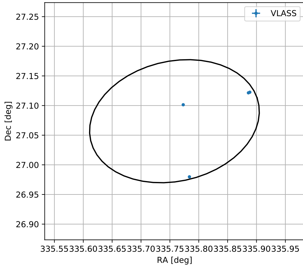
4FGL J2223.0+2704
