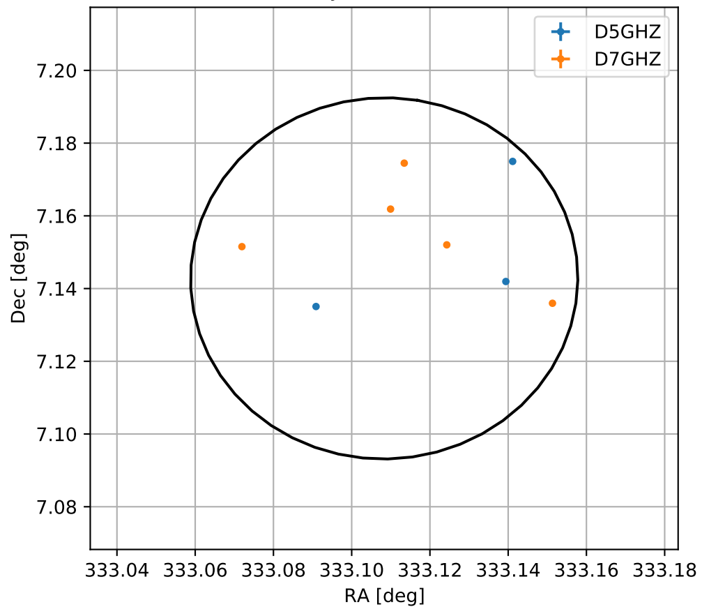
4FGL J2212.4+0708
