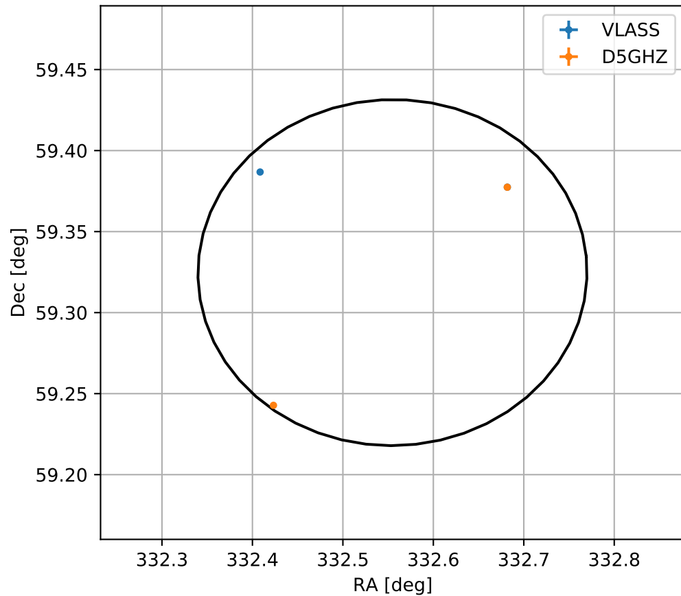
4FGL J2210.2+5919
