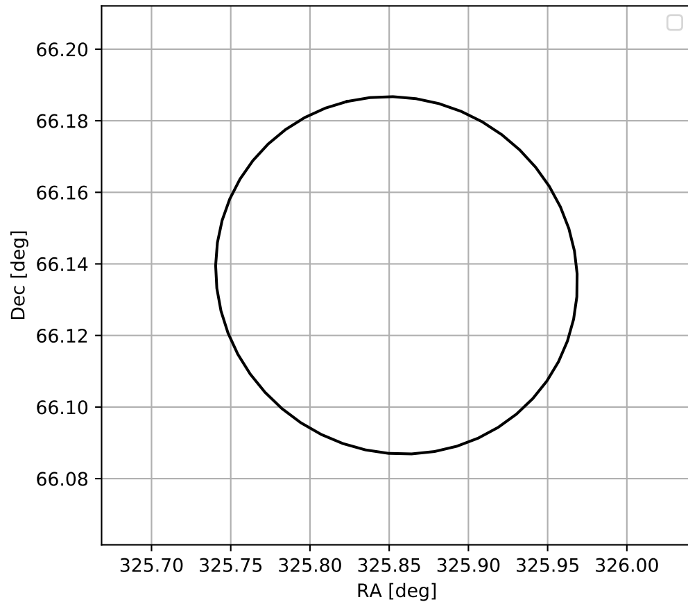
4FGL J2143.4+6608c
