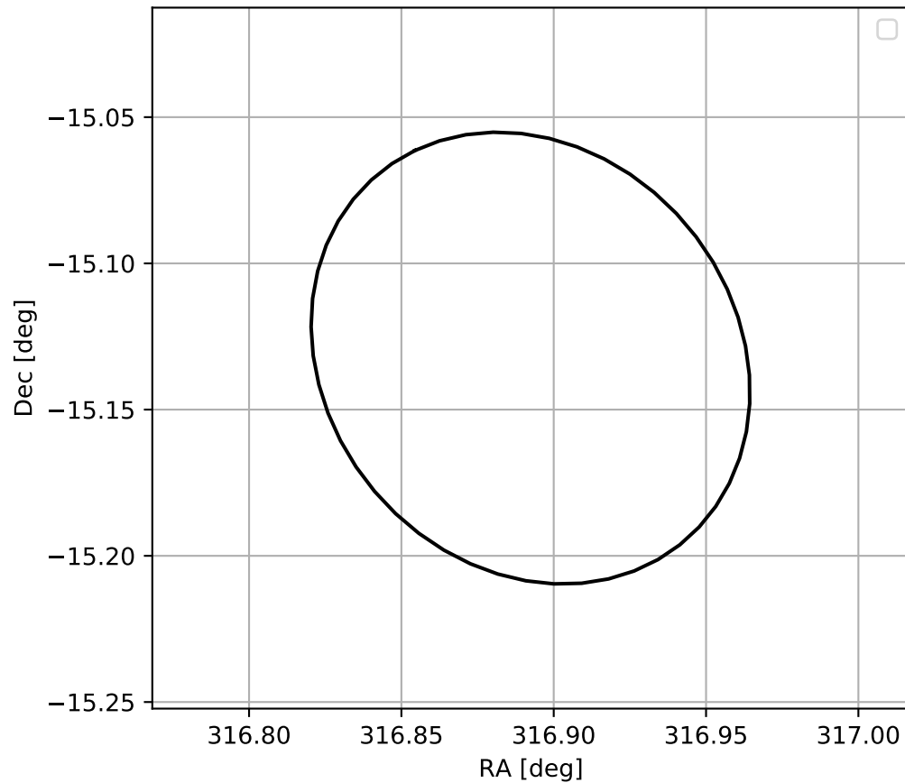
4FGL J2107.5-1507
