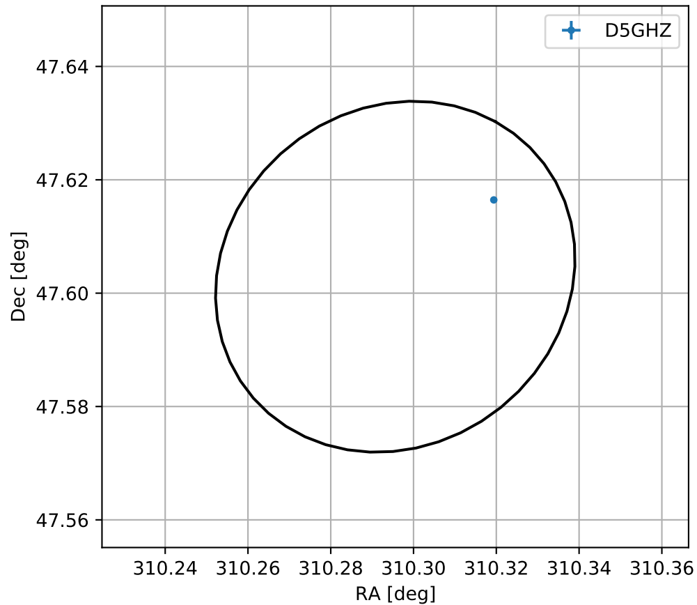
4FGL J2041.1+4736
