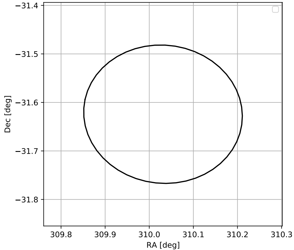
4FGL J2040.1-3137
