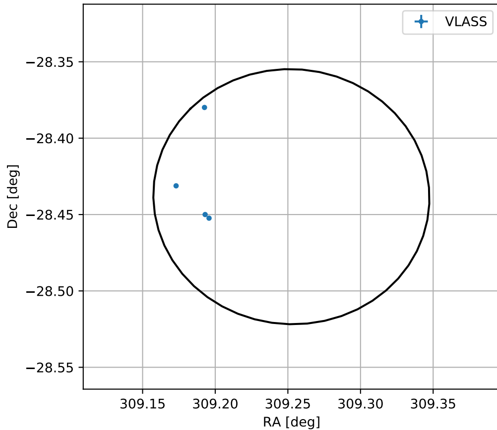
4FGL J2037.0-2826
