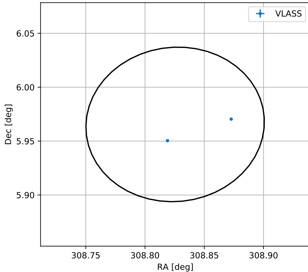
4FGL J2035.3+0557
