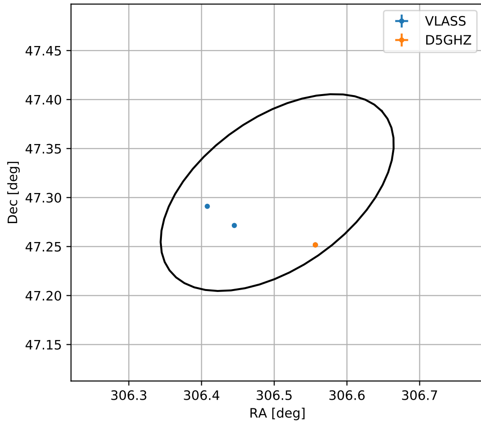
4FGL J2026.0+4718
