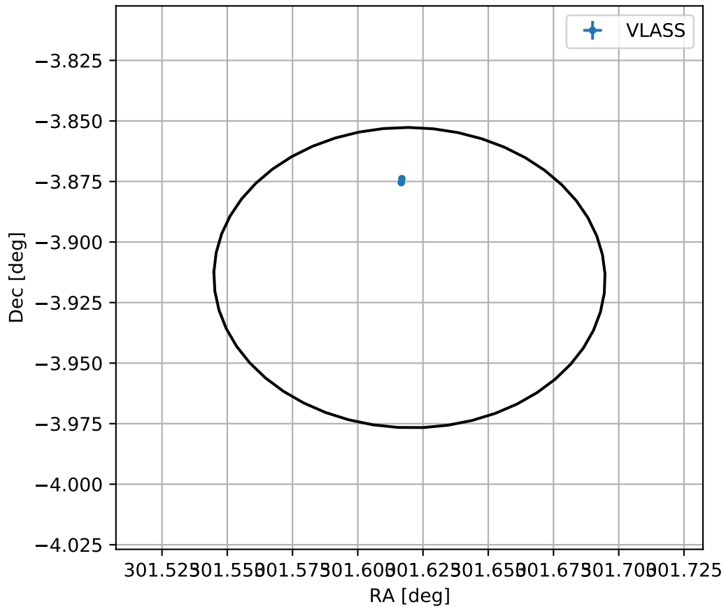
4FGL J2006.4-0354
