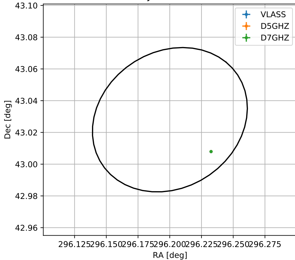
4FGL J1944.8+4301
