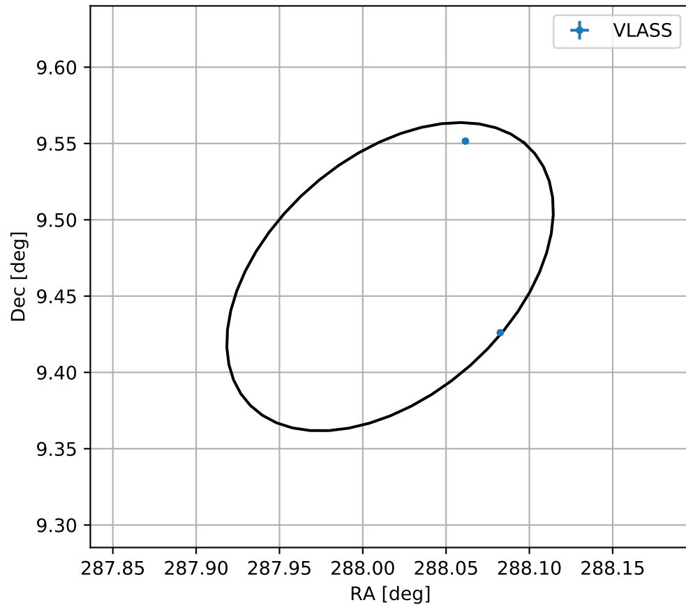
4FGL J1912.0+0927
