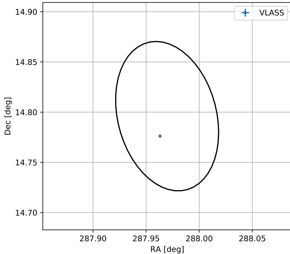
4FGL J1911.8+1447
