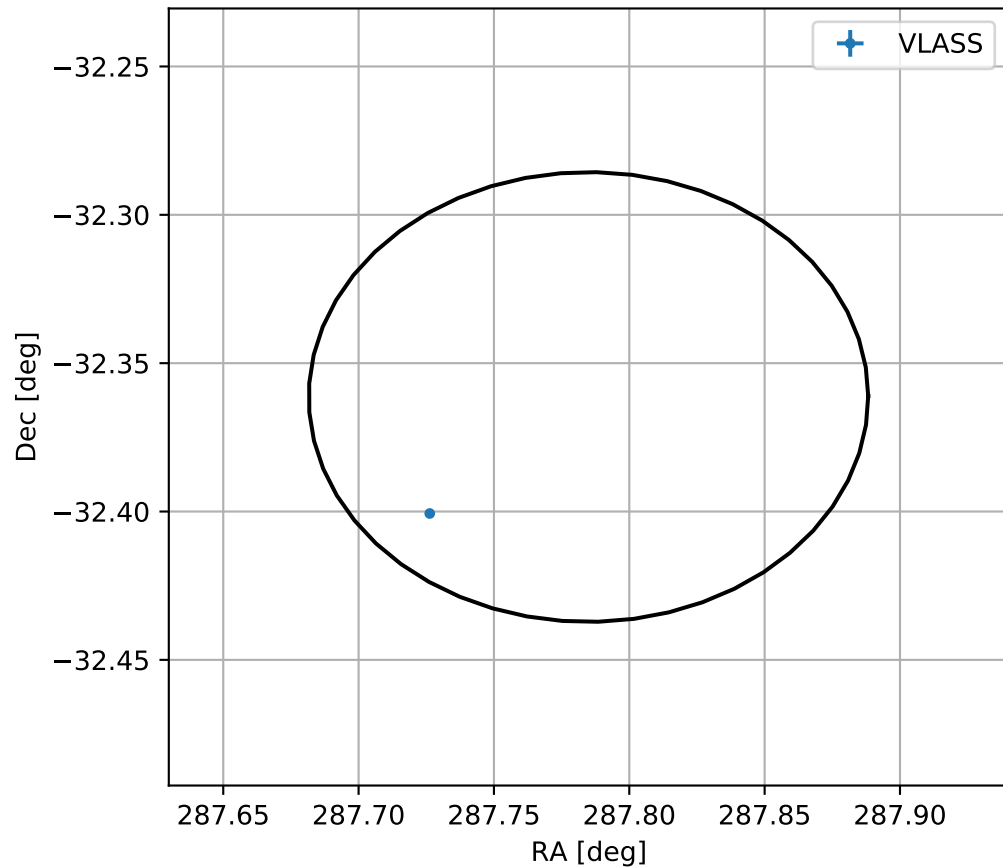
4FGL J1911.1-3221
