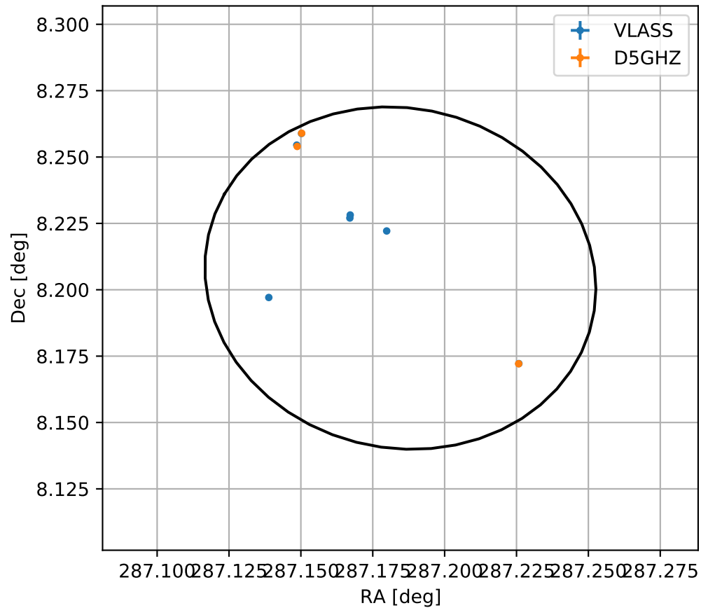
4FGL J1908.7+0812
