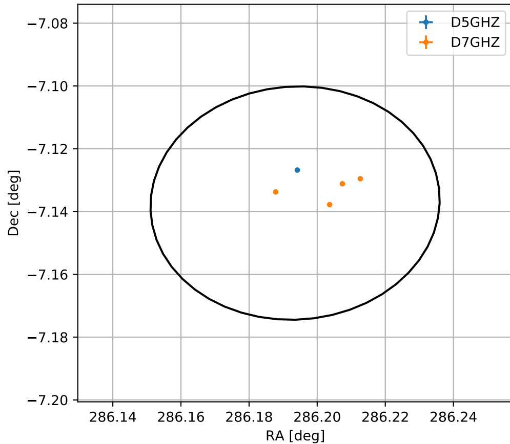
4FGL J1904.7-0708
