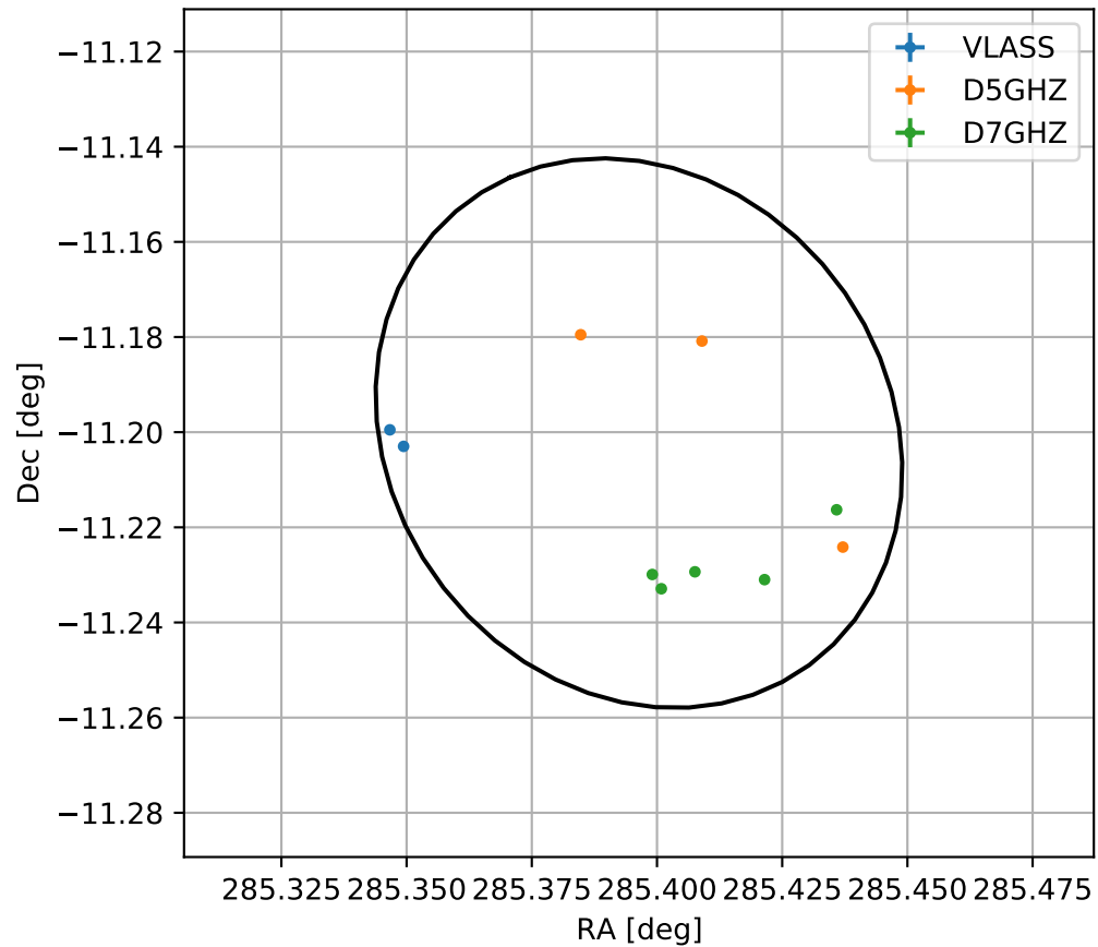
4FGL J1901.5-1112
