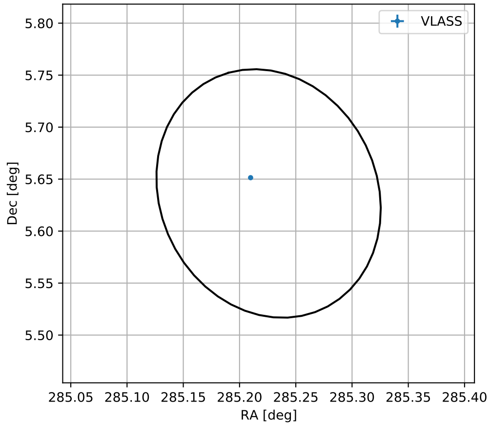
4FGL J1900.9+0538
