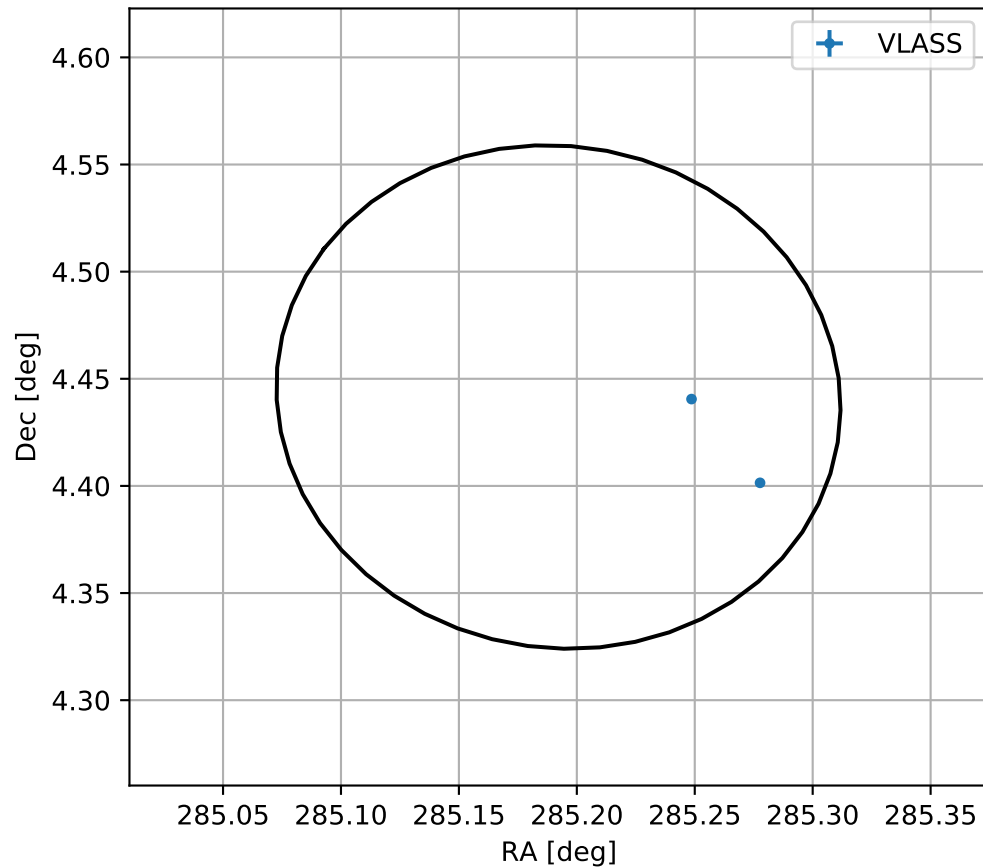
4FGL J1900.7+0426
