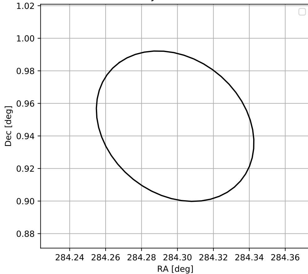
4FGL J1857.1+0056
