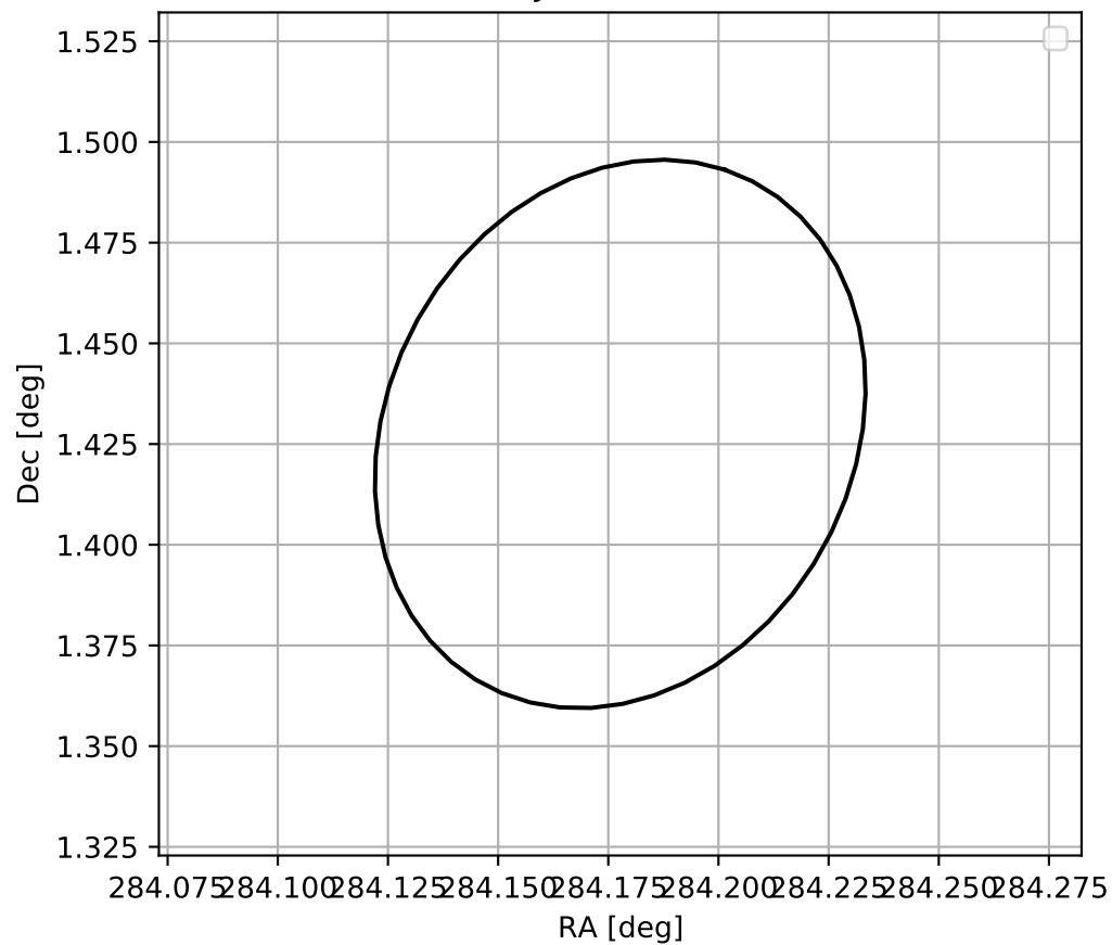
4FGL J1856.7+0125c
