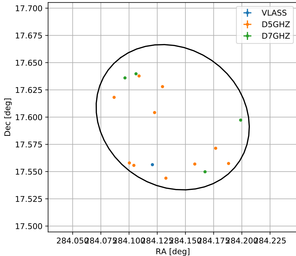
4FGL J1856.5+1735
