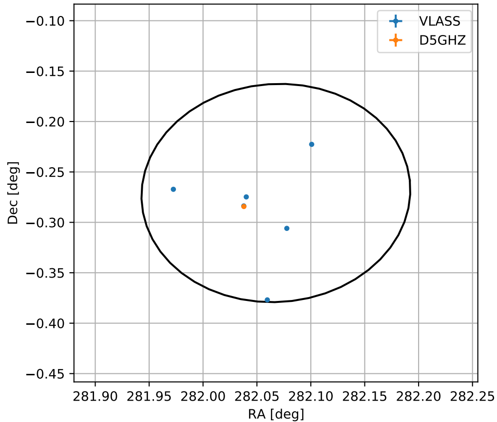
4FGL J1848.2-0016
