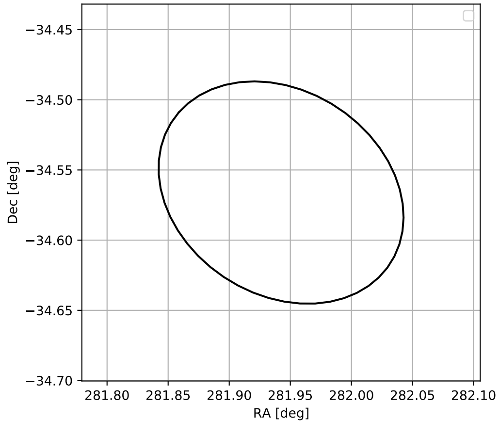
4FGL J1847.7-3433
