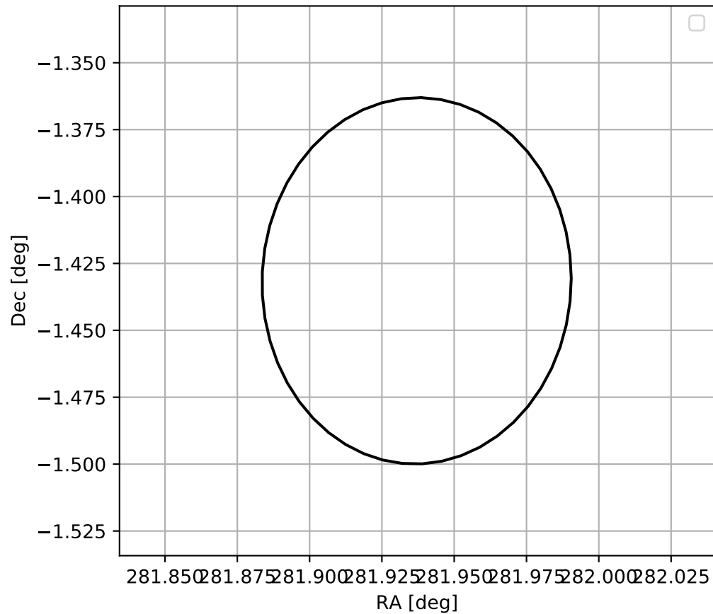
4FGL J1847.7-0125
