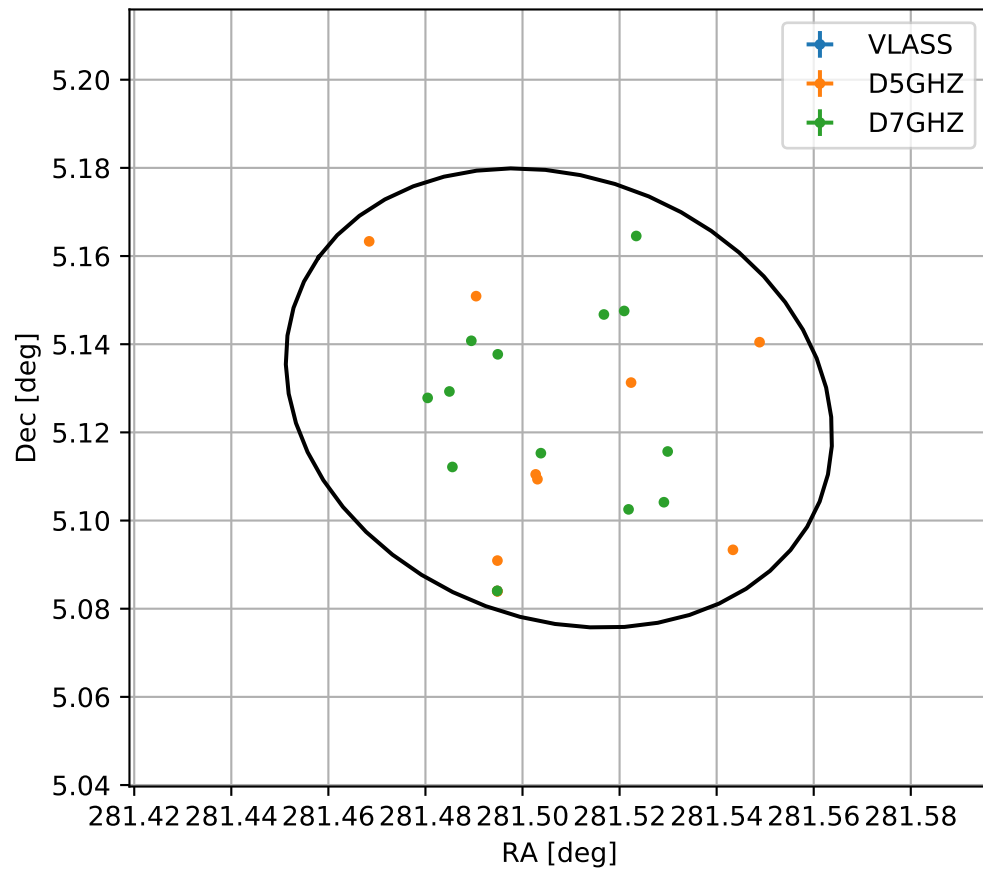
4FGL J1846.0+0507
