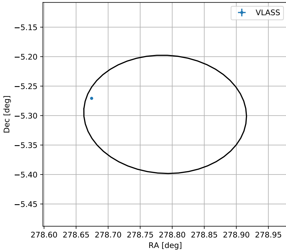
4FGL J1835.1-0517
