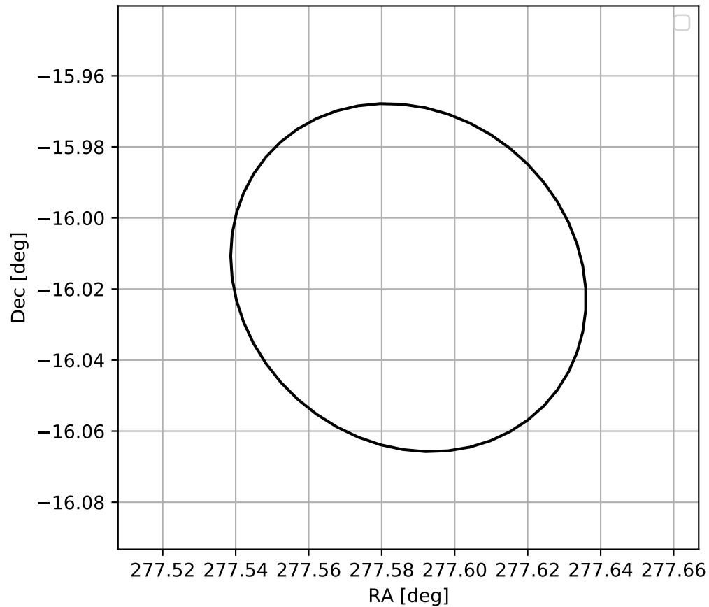
4FGL J1830.3-1601
