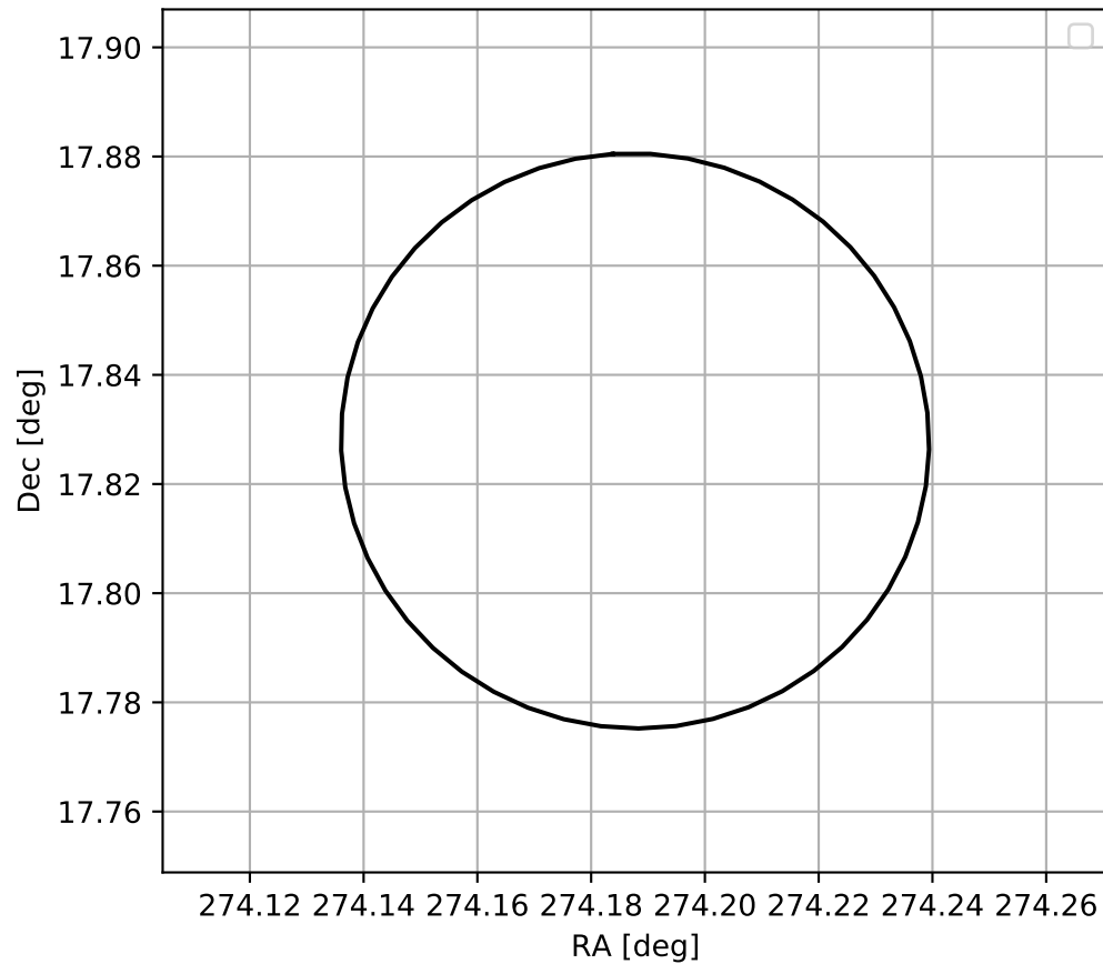
4FGL J1816.7+1749
