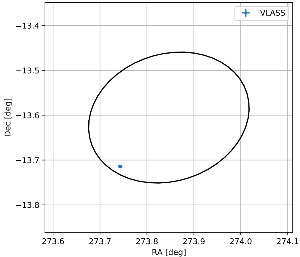
4FGL J1815.3-1336
