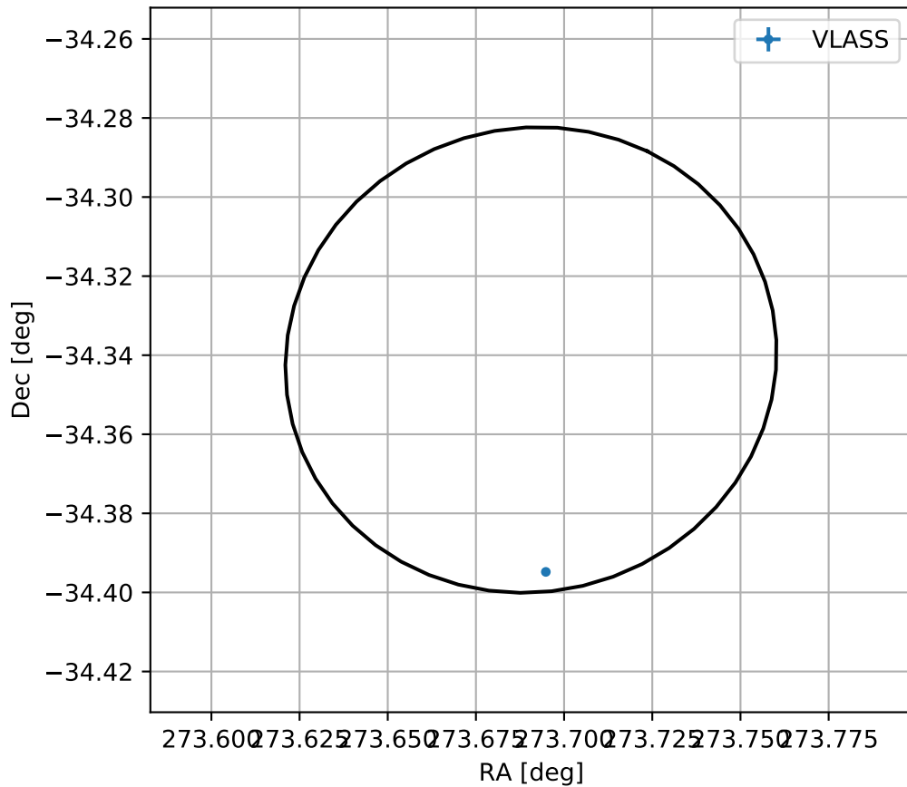
4FGL J1814.7-3420
