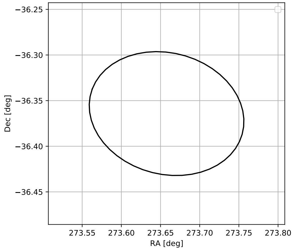
4FGL J1814.6-3621
