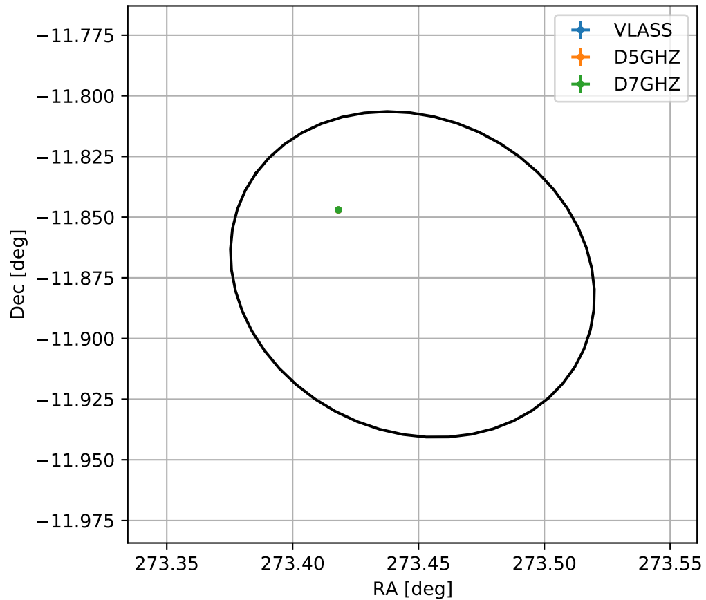
4FGL J1813.7-1152
