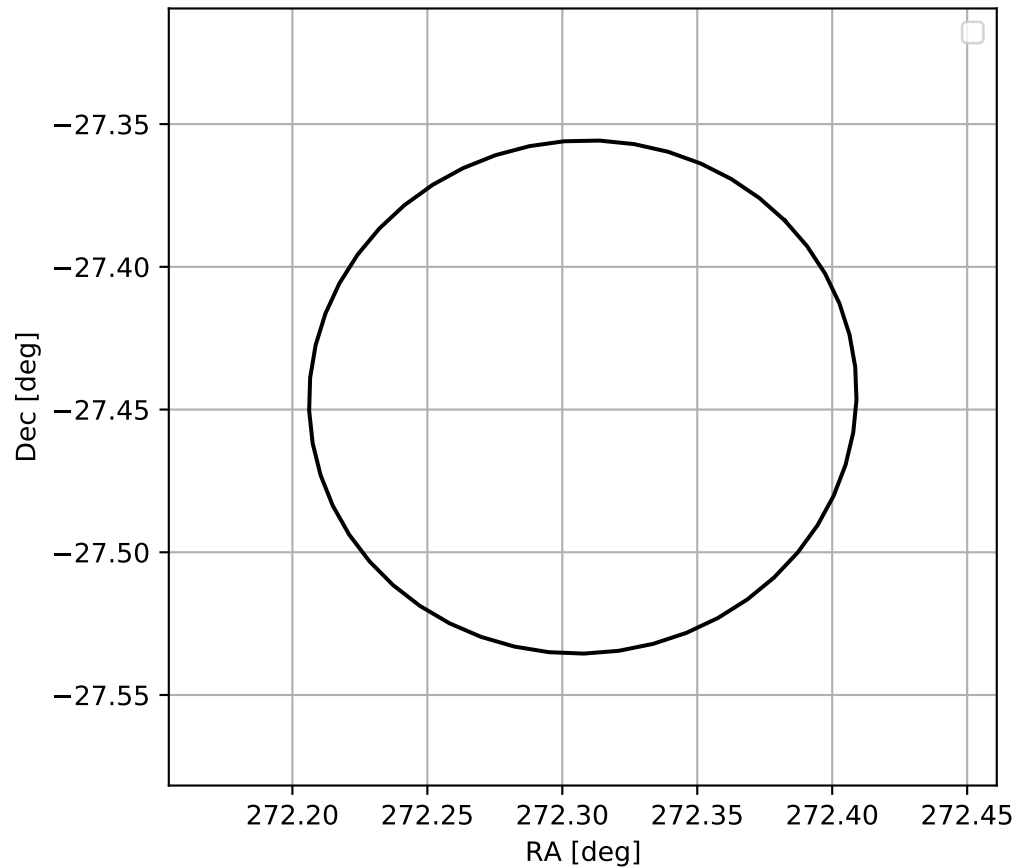
4FGL J1809.2-2726
