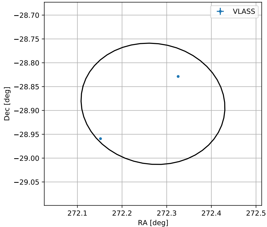
4FGL J1809.0-2853
