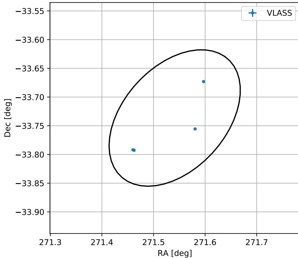
4FGL J1806.1-3344
