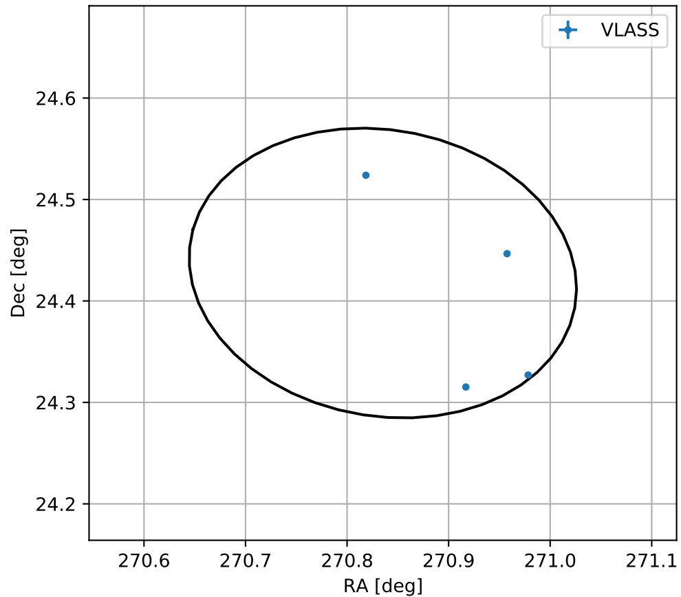
4FGL J1803.3+2425
