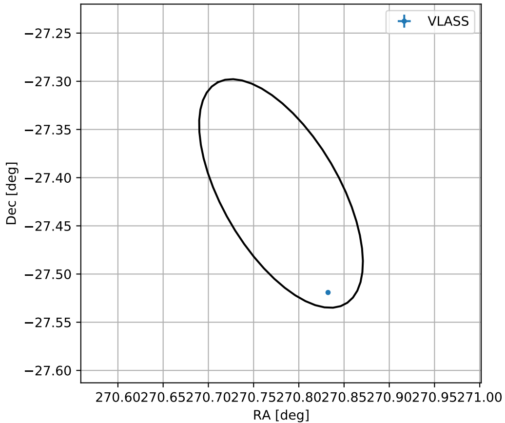
4FGL J1803.1-2724
