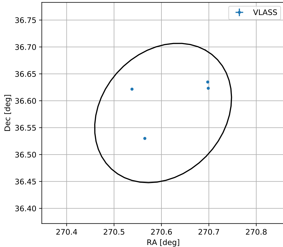
4FGL J1802.4+3634
