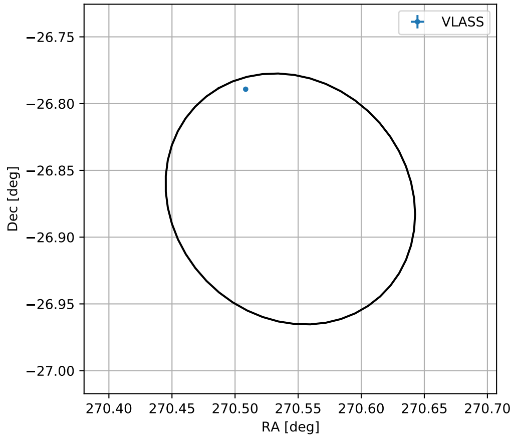
4FGL J1802.1-2652
