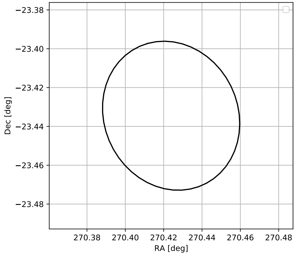
4FGL J1801.6-2326
