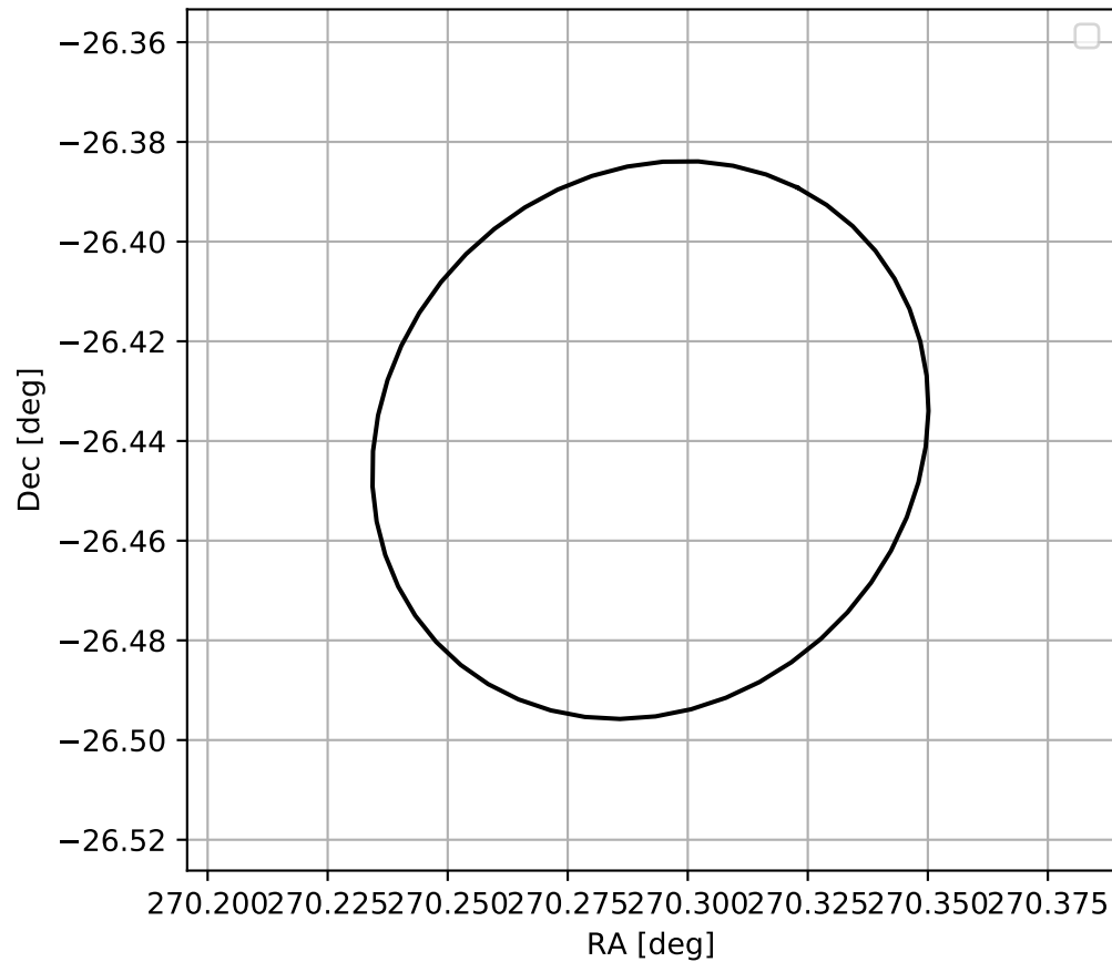
4FGL J1801.1-2626
