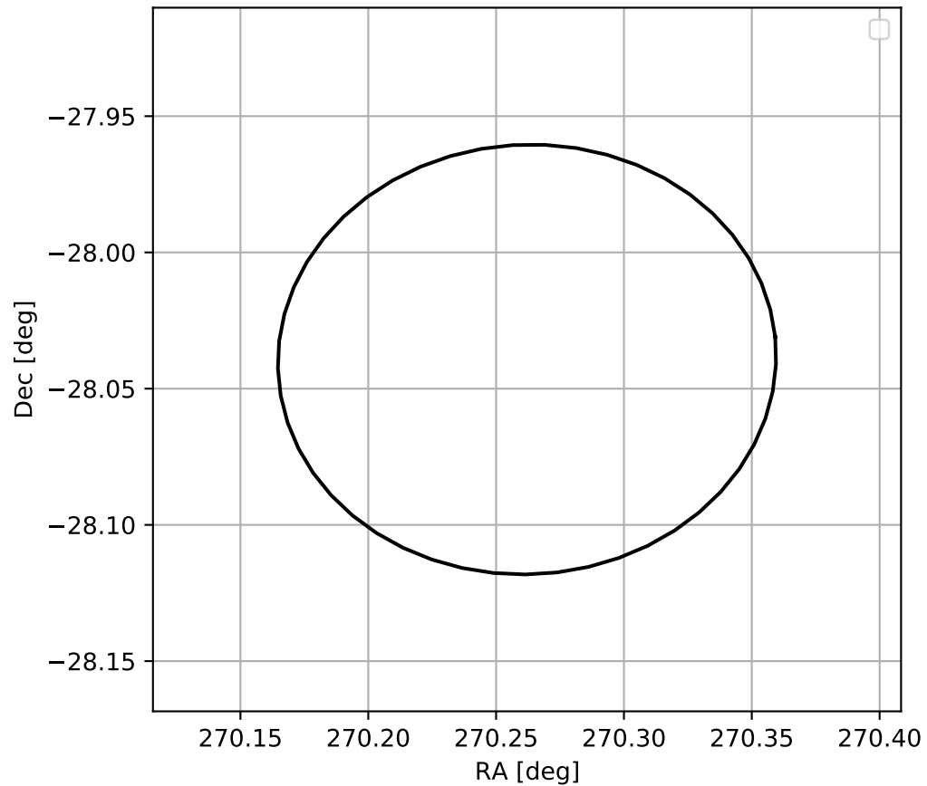
4FGL J1801.0-2802
