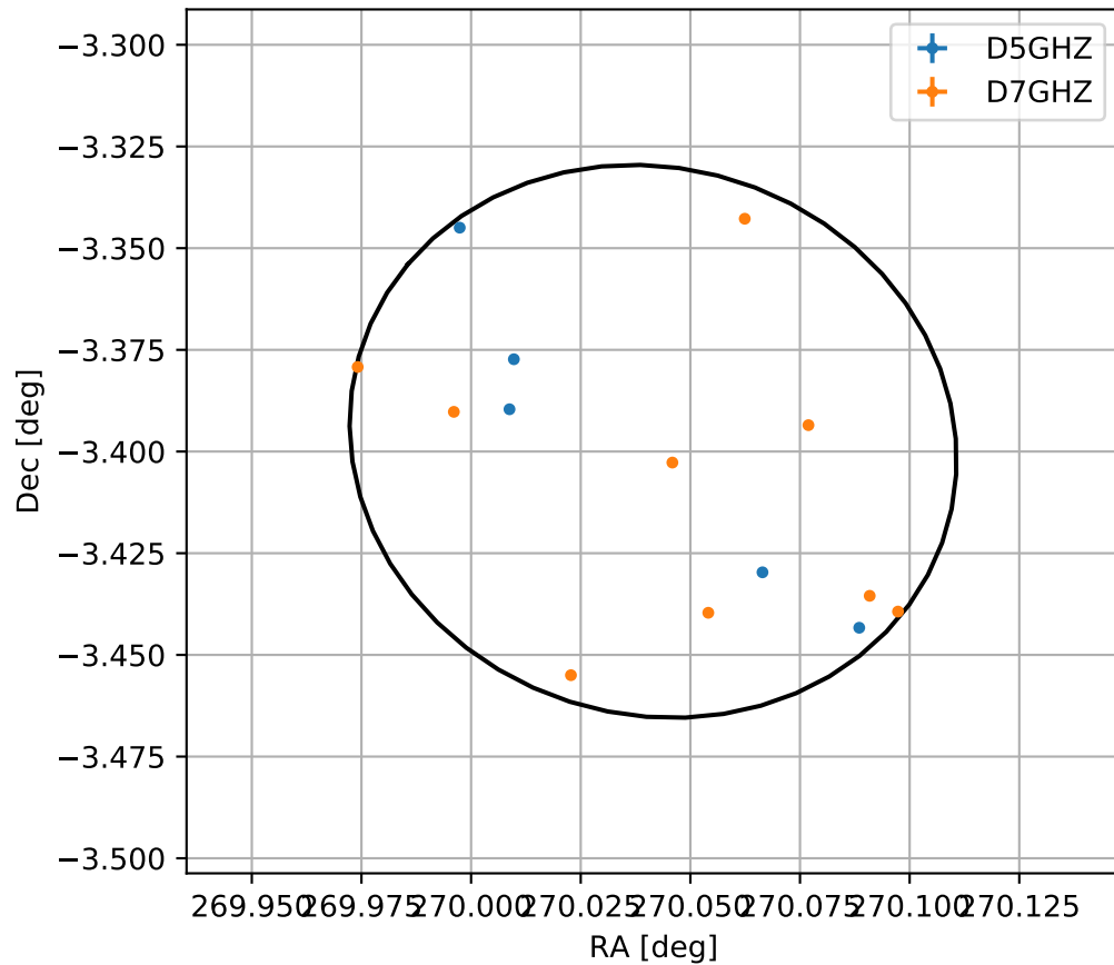
4FGL J1800.1-0323
