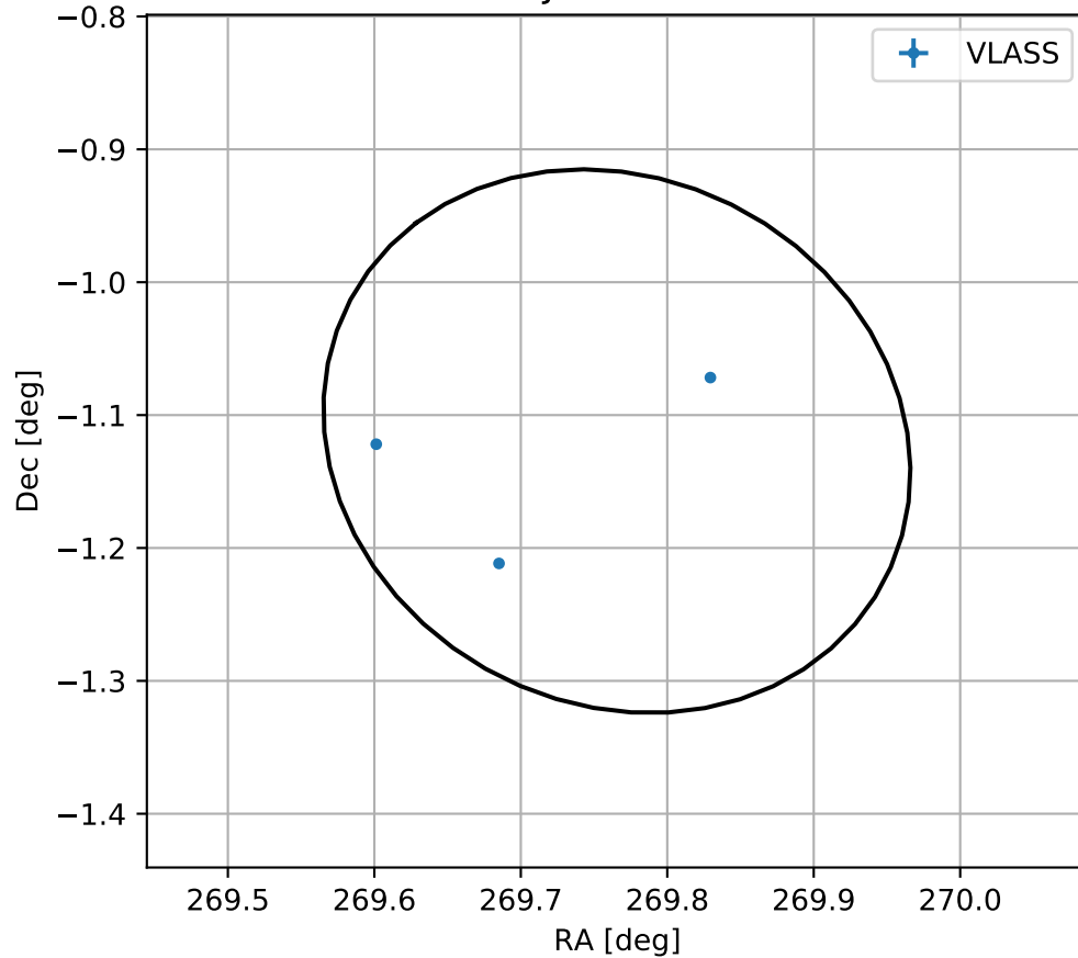
4FGL J1759.0-0107
