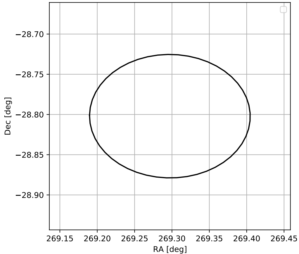
4FGL J1757.1-2848c
