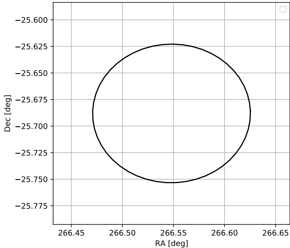
4FGL J1746.1-2541
