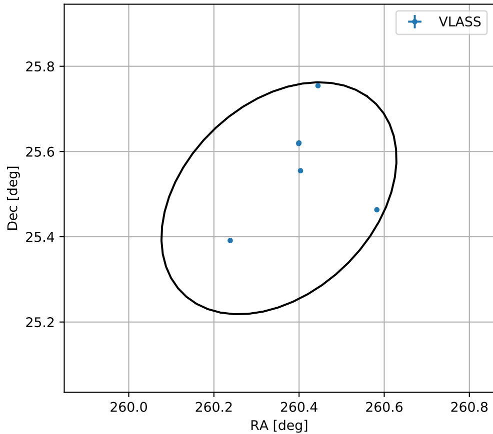
4FGL J1721.4+2529
